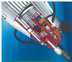
セラミック製4連アクシャルピストンポンプ
